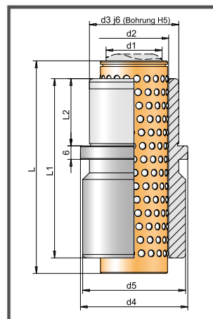
Zeichnung zu N 063.
