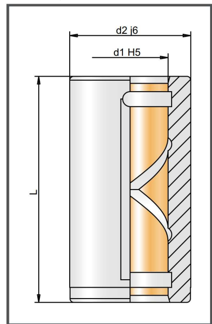
Zeichnung zu N 9047.
