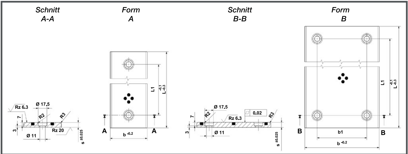
Zeichnung zu 5130.
