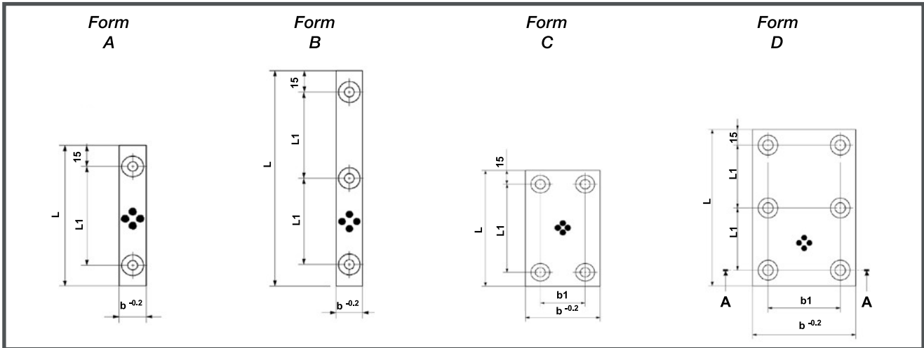
Zeichnung zu 5132.
