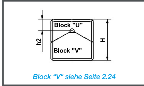
Zusammengebauter Zustand 5165. + 5165.1.
