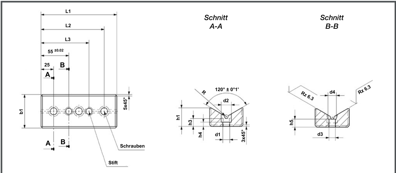
Zeichnung zu 5165.1.
